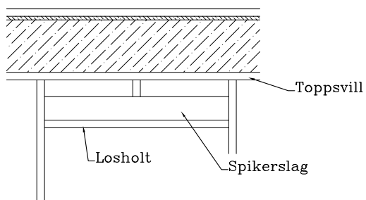
Fig 2. Vindusåpning med spikerslag for beslag. Spikerslaget kan også fungere som bæring for mindre laster.
