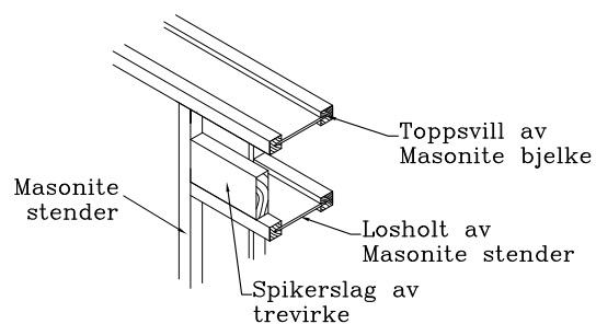
Fig 3. Utsnitt av fig 2 med spikerslag/bæring av trevirke.
