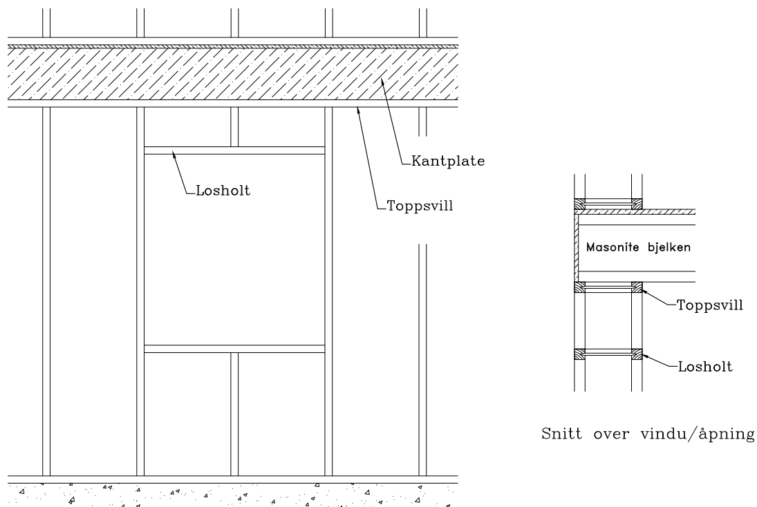
Fig 1. Vindusåpning uten bæring over losholt.
